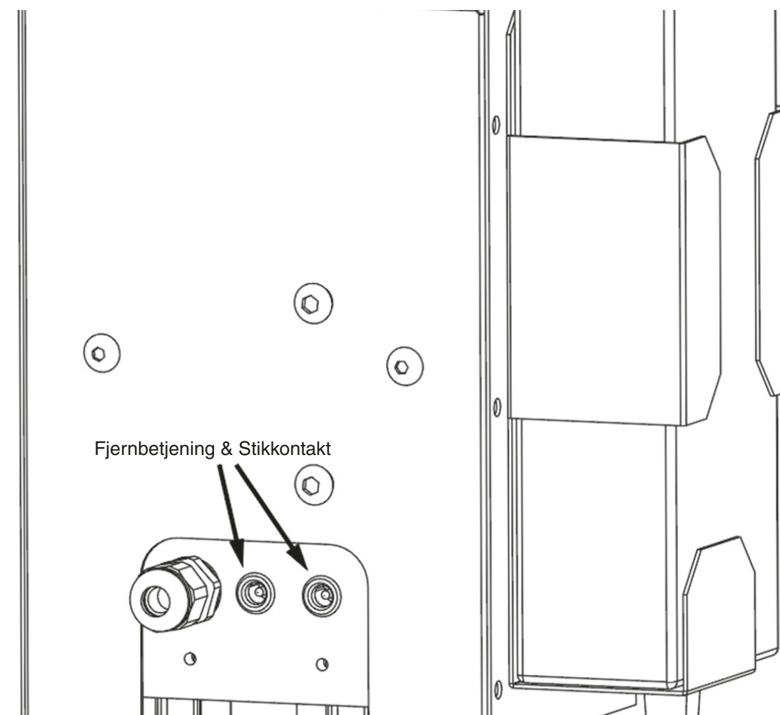
Figur 4: Øverste strømstik og strømforsyningsbeslag
