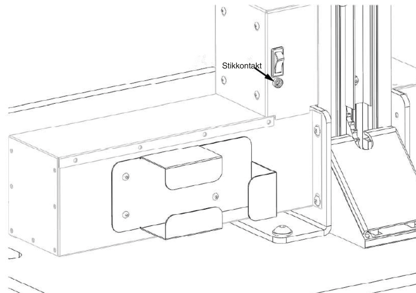
Figur 5: Nederste strømstik og strømforsyningsbeslag
